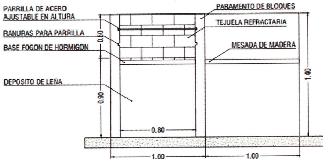
2 DETALLE PARRILLA
